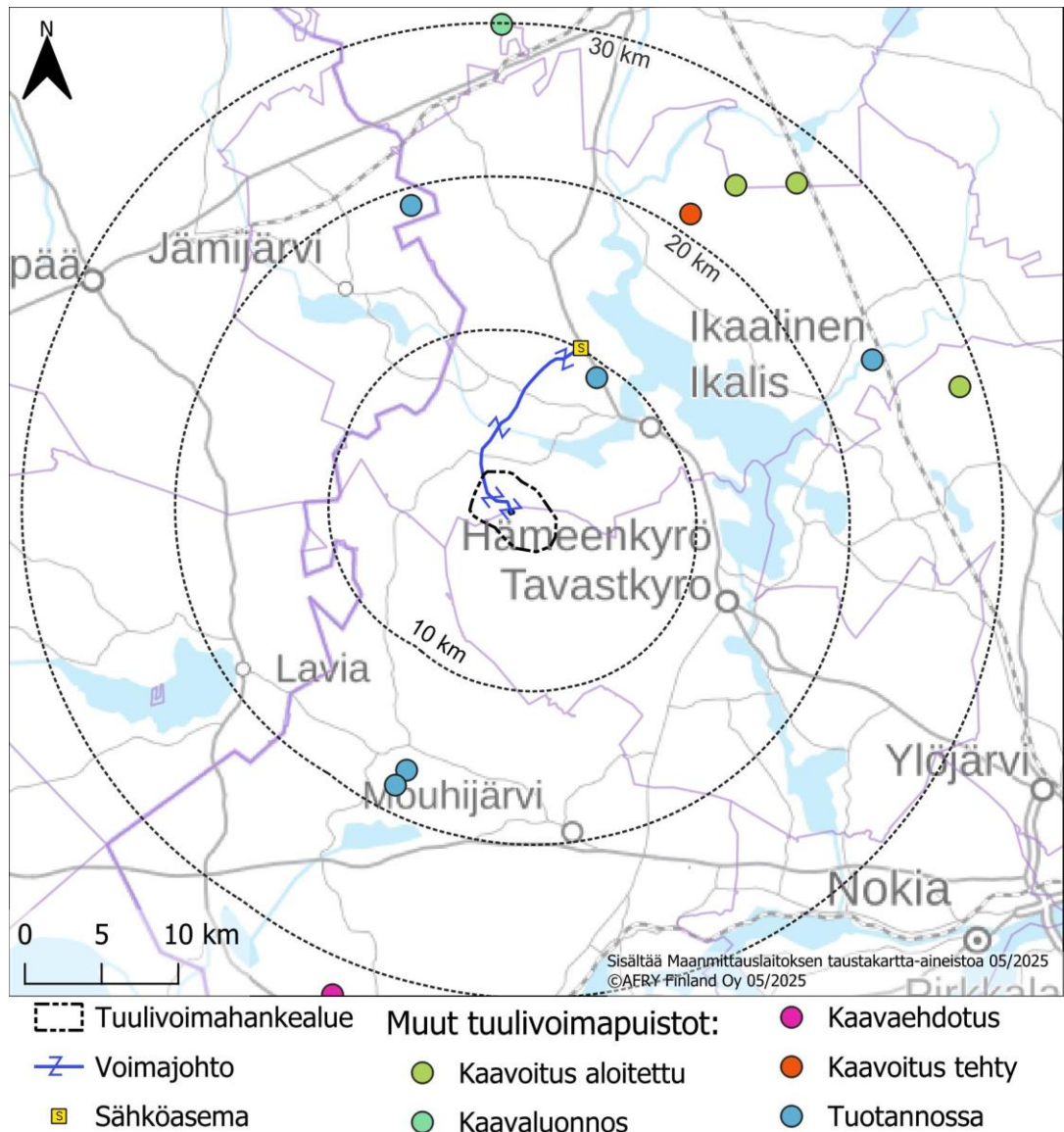
Kuva 6-1. Lähialueen tuulipuistohankkeet.
