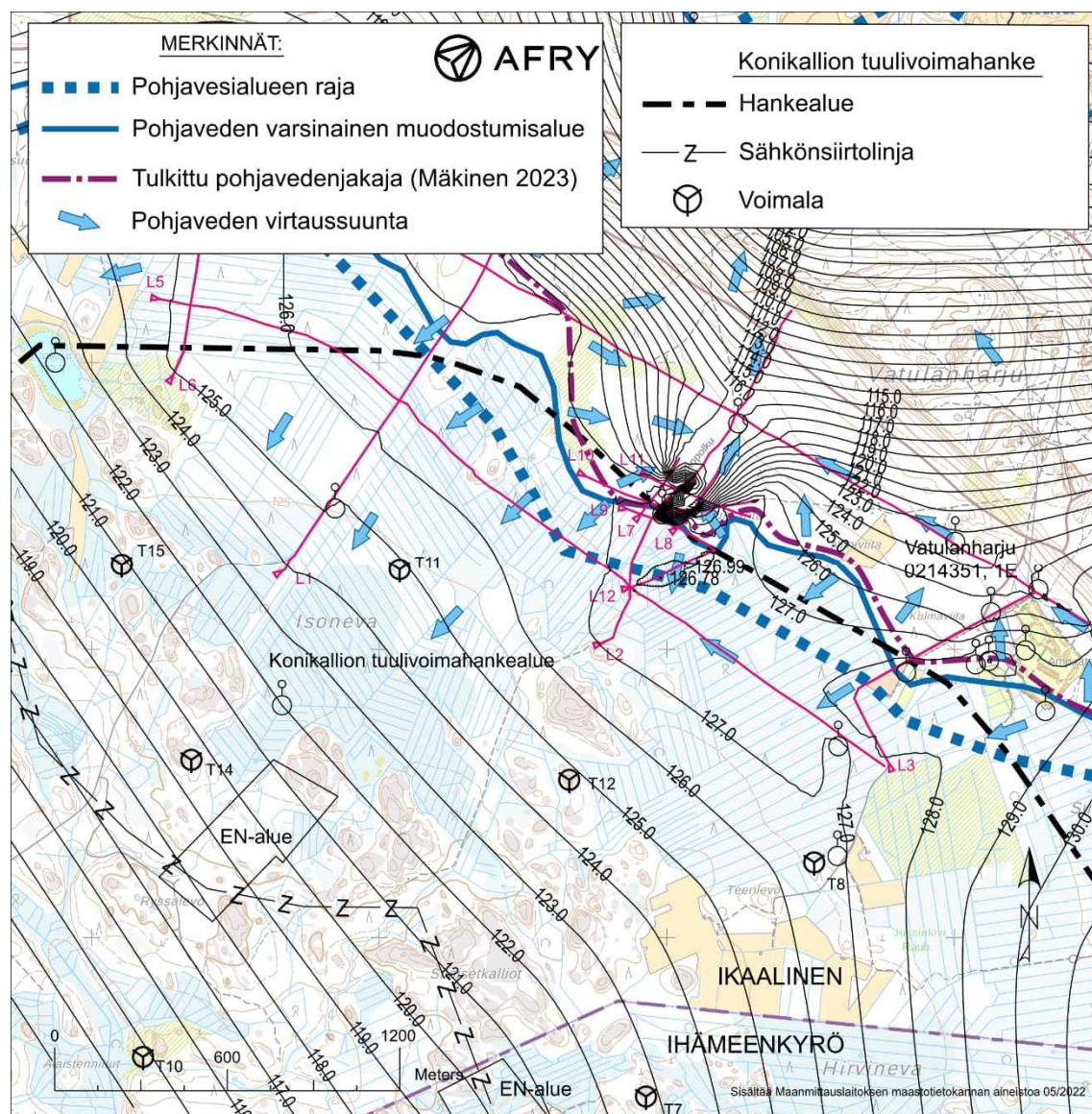
Kuva 4. Pohjaveden pinnan sama-arvokäyrästöt. Kuva on laaijempana karttaliitteessä 4.
